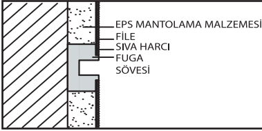
S - 39 DÜZ FUGA PROFİLİ
